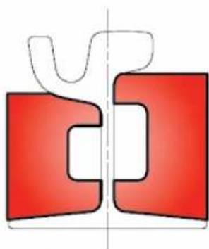
WERSJA 3 - "niskie" szyny: 60R1, 60R2, 59R1, 59R2
